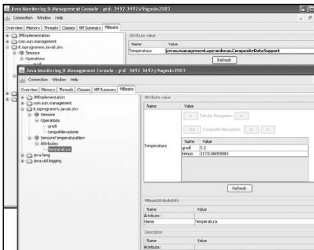
Figura 6.8: Proprietà temperatura
